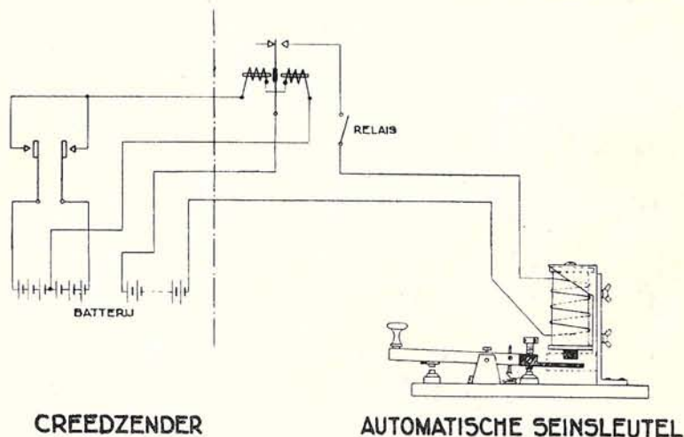
Fig. 4. Constructie- en schakelschema van den automatischen seinsleutel.
