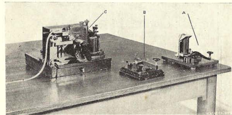
Fig. 3. Onderwijs-installatie voor 1 leerling. A. Automatische seinsleutel. B. Gewone seinsleutel. C. Morsetoestel.
