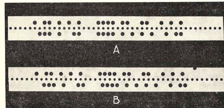
Fig. 2. Schrift, verkregen met de Creed-ponsdoos: A zooals het wordt geproduceerd, B zooals het moet worden gelezen.
